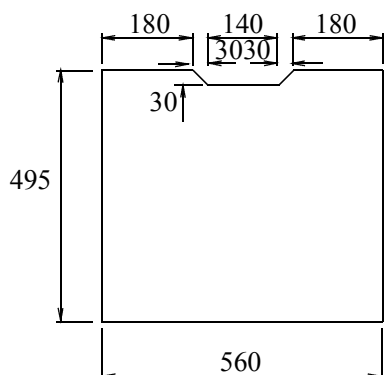
ソケット 450 用ふた 560 × 120 × 495 80kg
