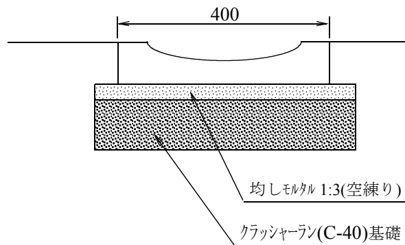
施工断面図
