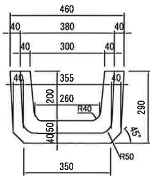
断面図 B-B
