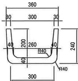
断面図 C-C
