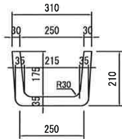
断面図 C-C
