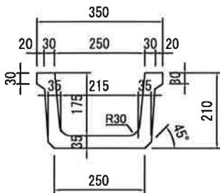
断面図 B-B
