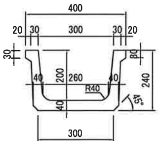
断面図 B-B
