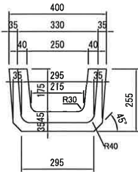
断面図 B-B
