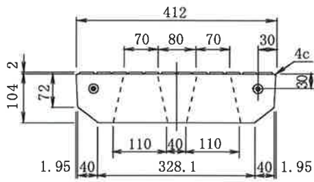
400用集水ふた
