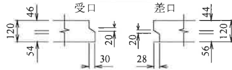
底板・側壁
