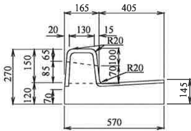
水抜型 L=2000 270 × 570 × 2000 参考重量 450kg
