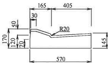
切下型 L=2000 170 × 570 × 2000 参考重量 386kg
