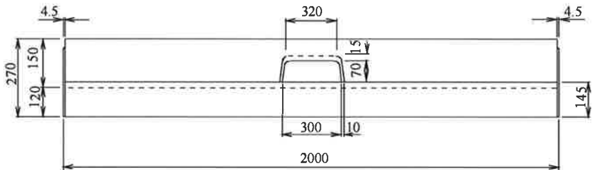
水抜型 L=2000 270 × 570 × 2000 参考重量 450kg
