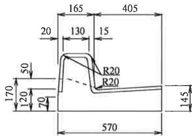
摺付型 L=2000 170/270 × 570 × 2000 参考重量 447kg
