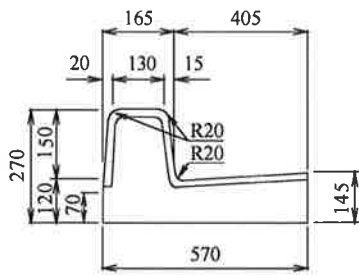
標準型 L=2000 270 × 570 × 2000 参考重量 457kg
